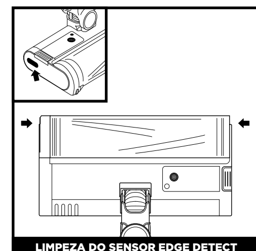
LIMPEZA DO SENSOR EDGE DETECT
