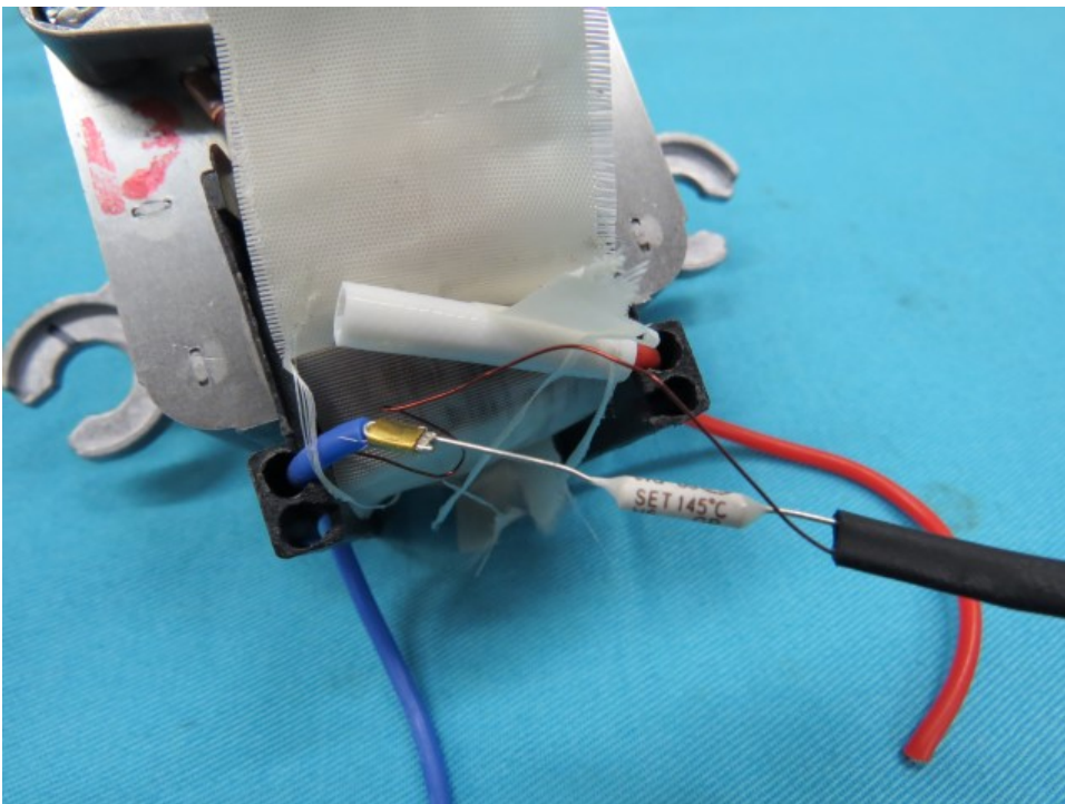
View of Fan Motor Thermal Fuse
