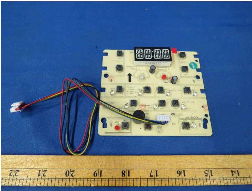
UI PCBA
