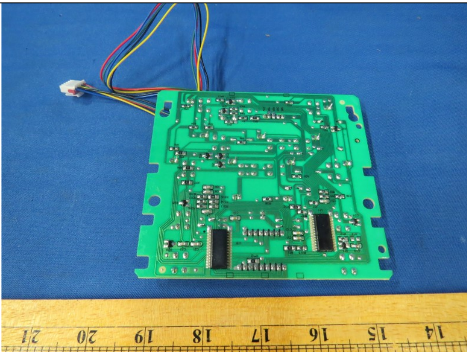
UI PCBA
