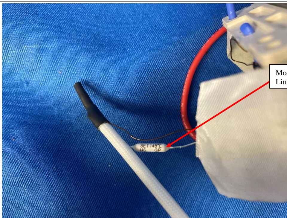
Motor Thermal Link
